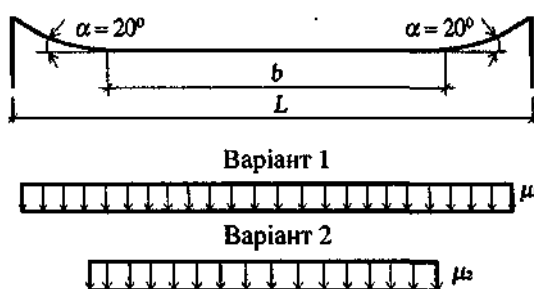
Схема 12. Висячі покриття циліндричної форми
