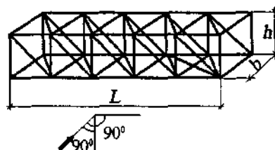
Схема 18. Ґратчасті вежі та просторові ферми
